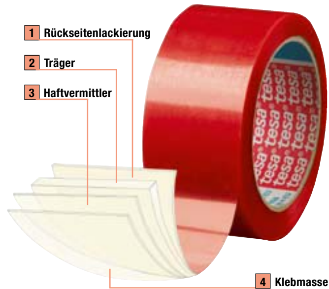
Aufbau eines einseitig klebenden Klebebandes
