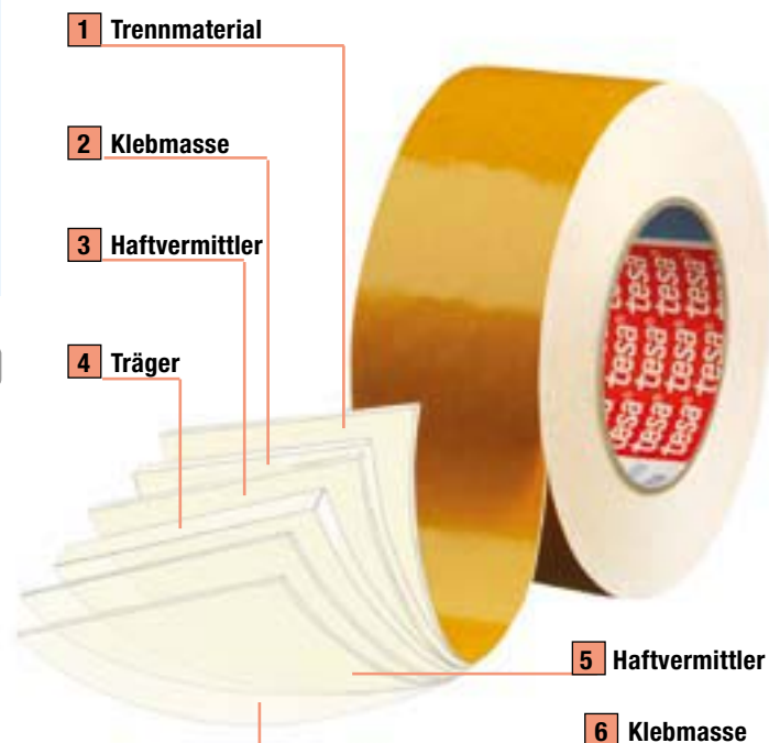
Aufbau eines doppelseitig klebenden Klebebandes
